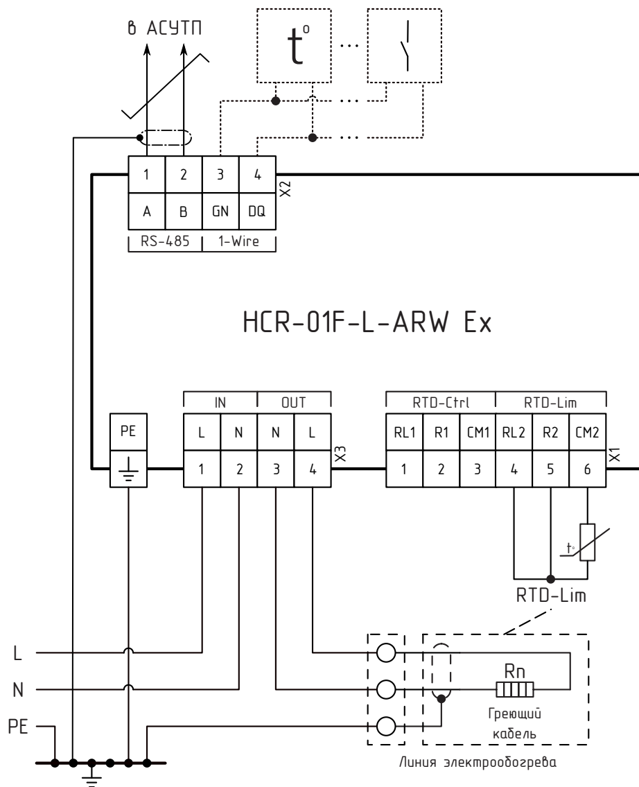
Рисунок В.6 – Схема подключения HCR-01F-L-ARW Ex. Режим работы по 1 датчику (RTD-Lim)
