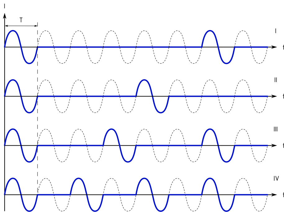
Рисунок 1.6 – Режим «Плавный пуск»
