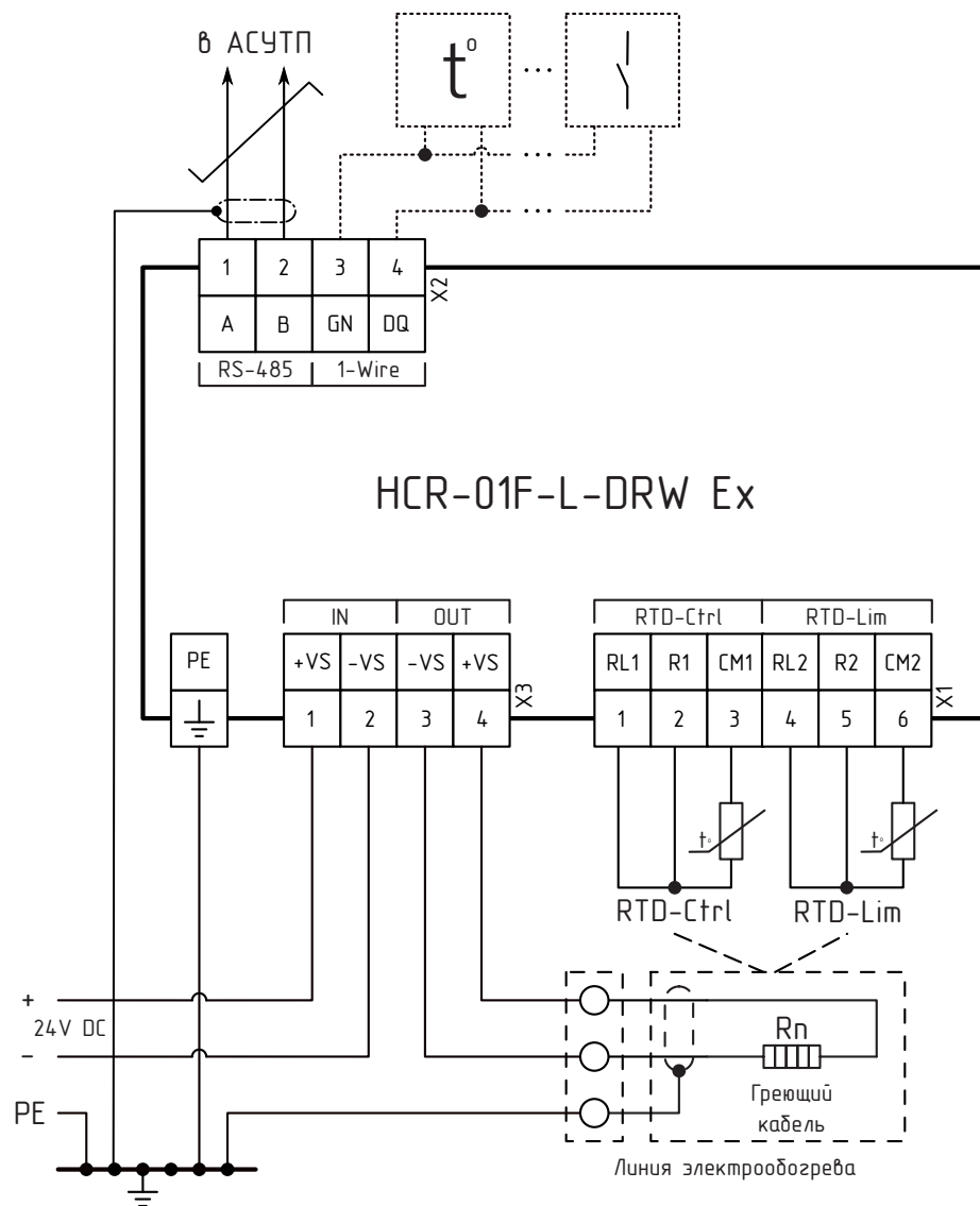
Рисунок В.4 – Схема подключения HCR-01F-L-DRW Ex
