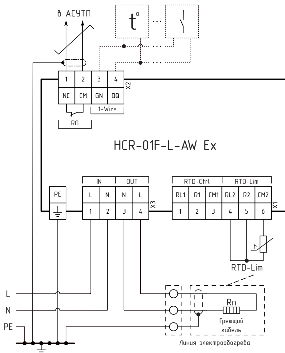
Рисунок В.5 – Схема подключения HCR-01F-L-AW Ex. Режим работы по 1 датчику (RTD-Lim)
