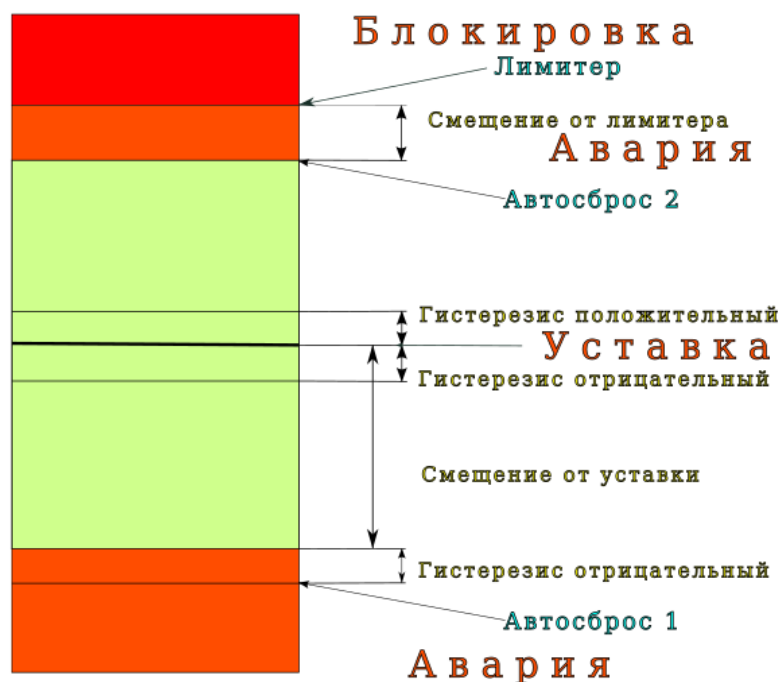
Рисунок 1.5 – Механизмы автосброса
