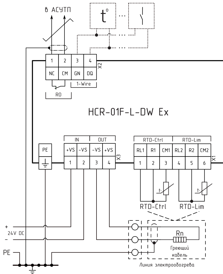
Рисунок В.2 – Схема подключения HCR-01F-L-DW Ex
